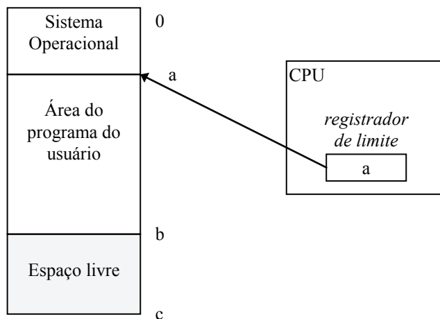
Figura 16 - Proteção de memória em sistemas monousuário usando registrador de limite.
