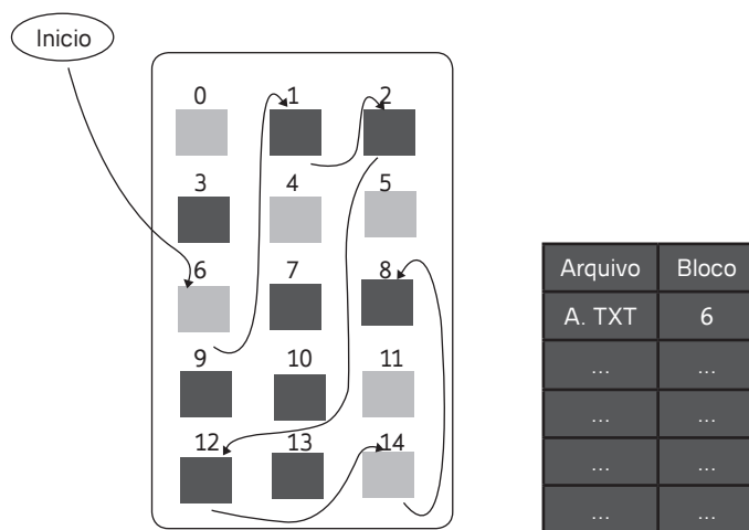
Fig. 24 - Alocação encadeada.
