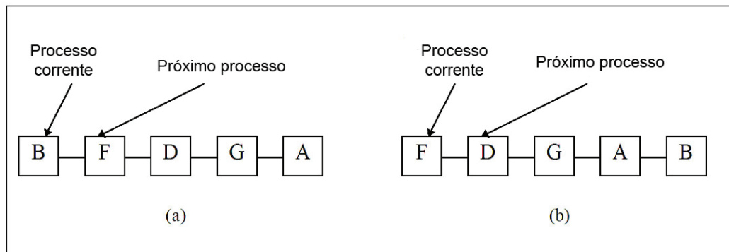
Figura 5 - Escalonamento Round Robin. (a) Lista de processos a executar. (b) Lista de processos a executar depois de terminado o quantum de 'B'.
