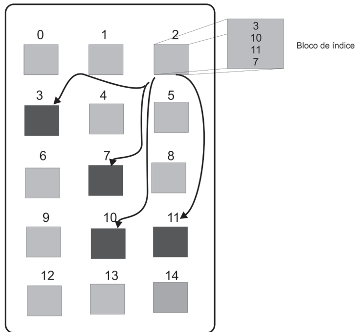
Fig. 25 - Alocação indexada.
