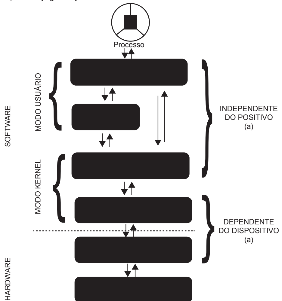
Fig. 26 – Arquitetura de camadas da gerência de dispositivos.
