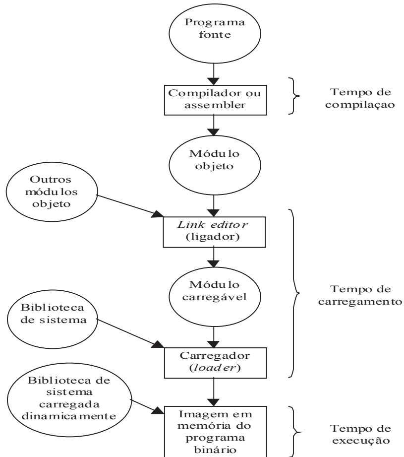
Figura 13 - Passos no processamento de um programa de usuário.
