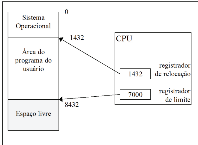
Figura 17 - Suporte do hardware para registradores de relocação e limite.
