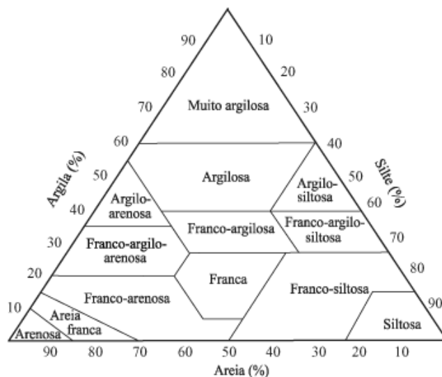
Triângulo de classificação textural de solos (Lemos e Santos, 1984).
